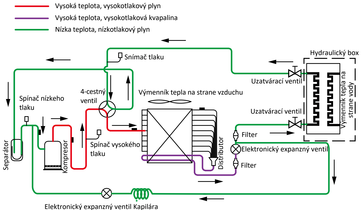
Obrázok 2-3.2: Tok chladiva počas prevádzky chladenia a rozmrazovania
