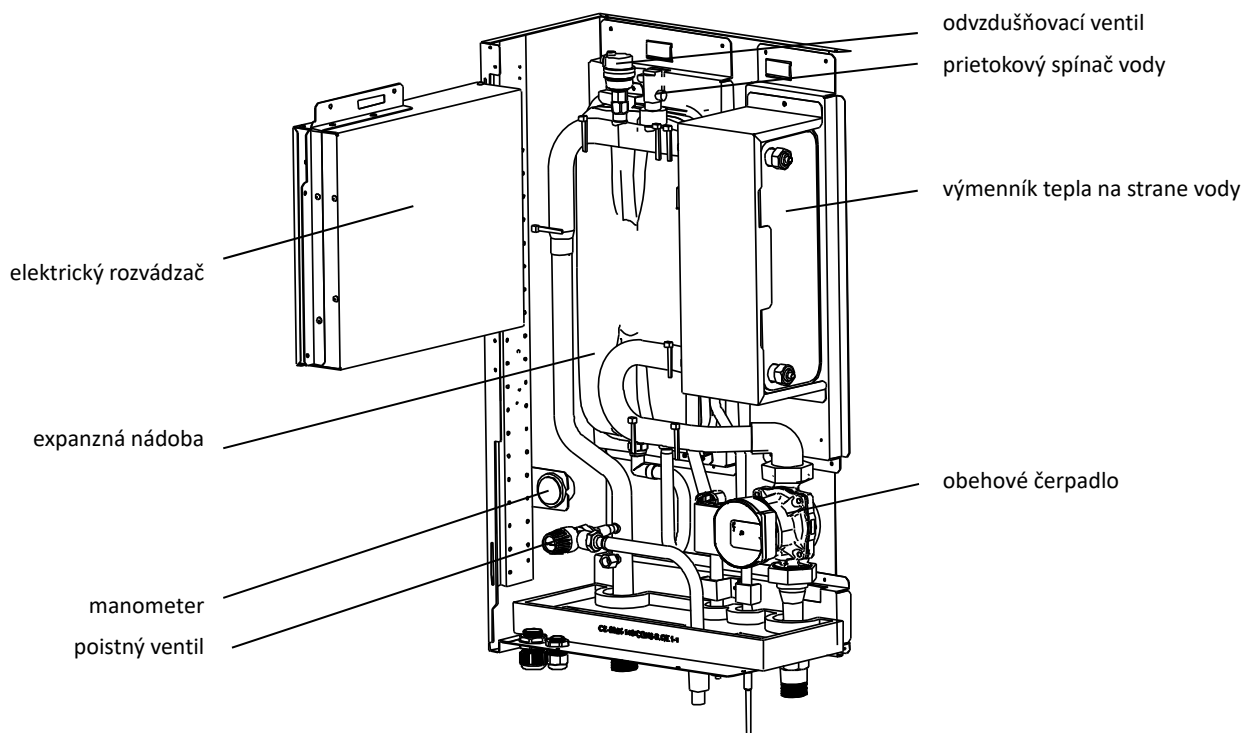
Obrázok 2-1.9: HOP60(100,160)WIDU(3), šikmý pohľad
