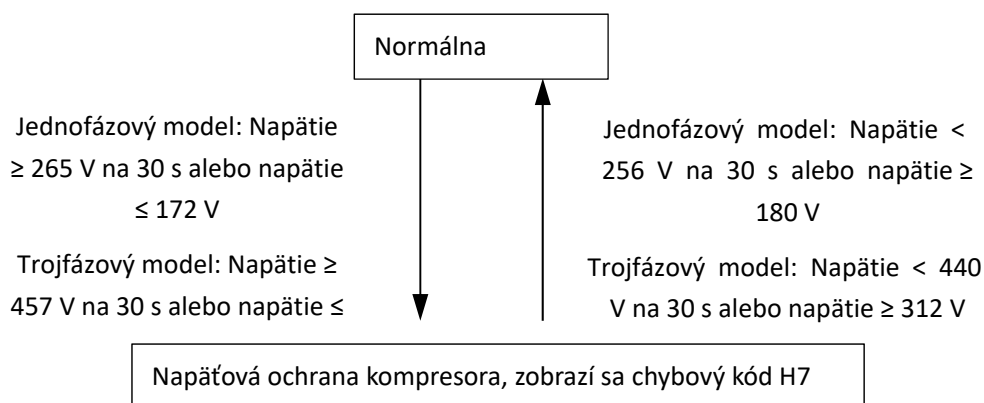
Obrázok 3-5.6: Riadenie napätvej ochrany kompresora
