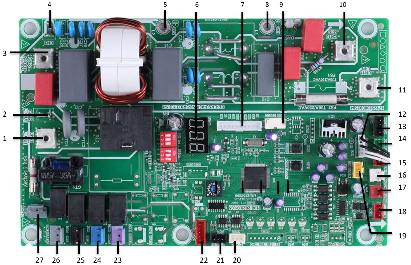
Obrázok 4-2.2: HOP4(6,8,10)WODU, hlavná PCB vonkajšej jednotky pre chladivový systém
