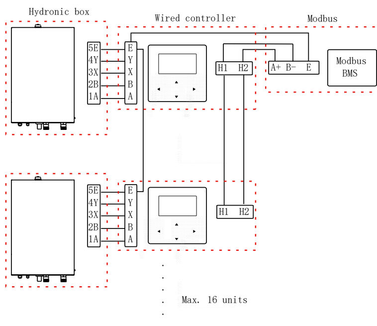
Obrázok 4-2.11: Zapojenie
