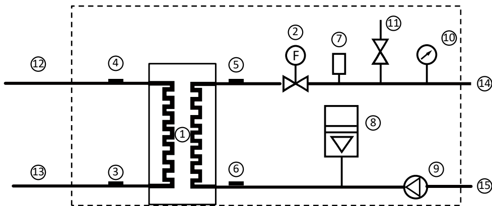
Obrázok 2-2.2: Schéma potrubných vedení hydraulického boxu
