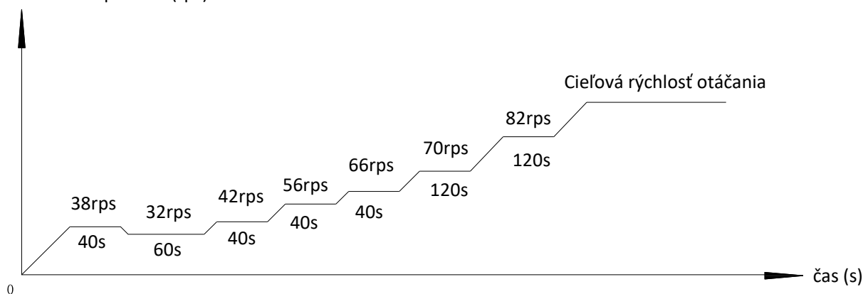
Obrázok 3-3.1: HOP4(6)WODU, program na spustenie kompresora 1 , keď je teplota vonkajšieho prostredia vyššia ako 3 °C
