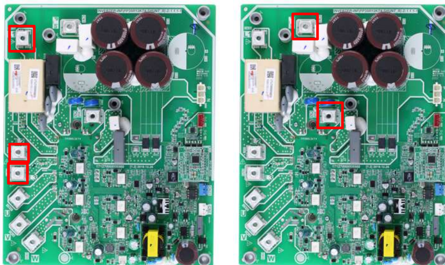
Obrázok 4-5.7: Zapojenie kábla DC zbernice (L1L2L3, PIN- POUT)
