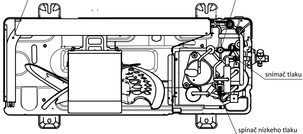
Obrázok 2-1.4: HOP8(10)WODU, pohľad spredu
