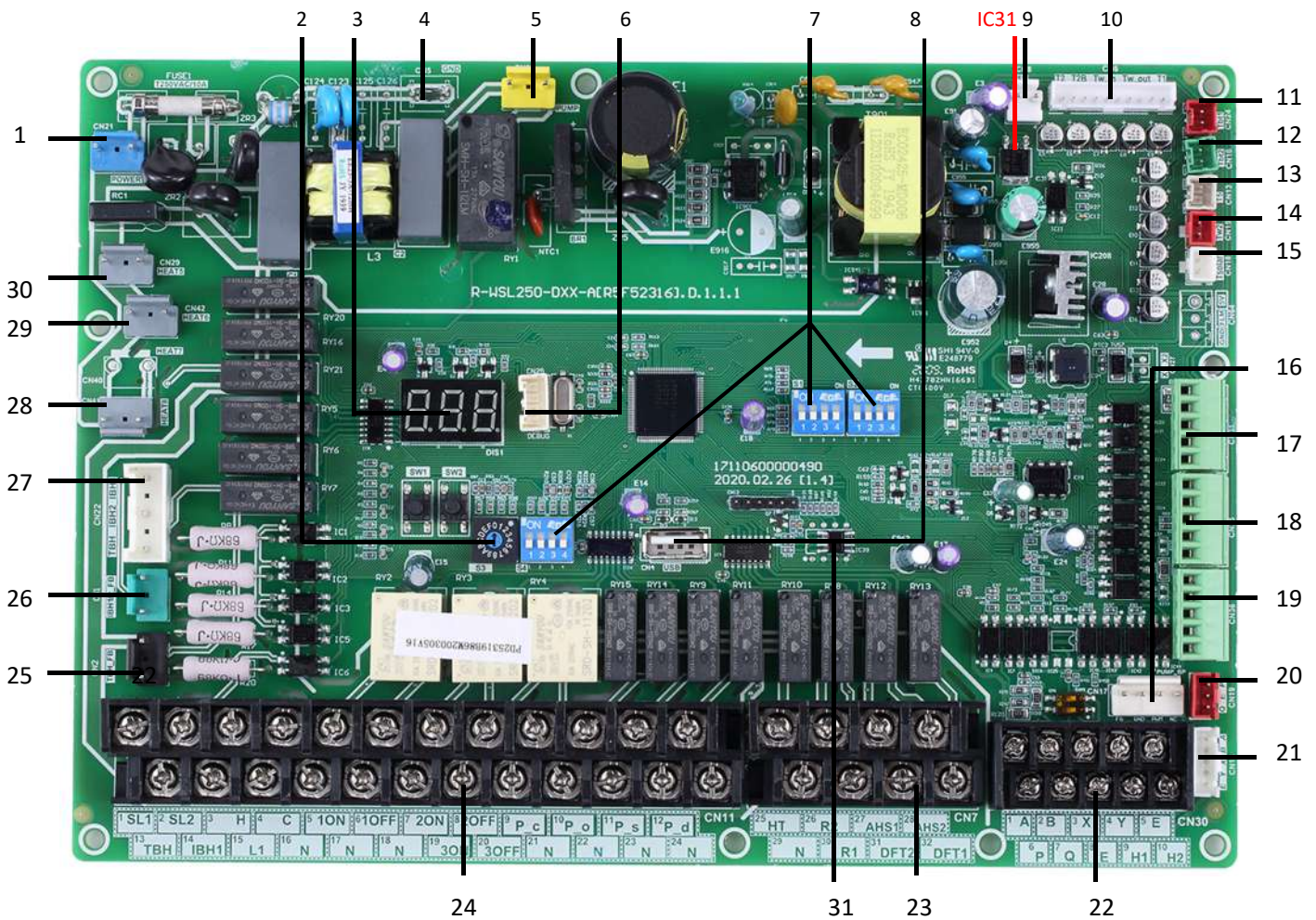
Obrázok 4-2.1: Hlavná PCB hydraulického boxu HOP60(100,160)WIDU(3)
