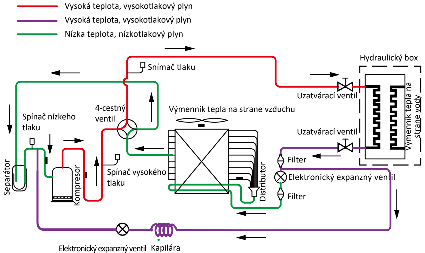
Obrázok 2-3.1: Tok chladiva počas prevádzky vykurovania alebo úžitkovej teplej vody
