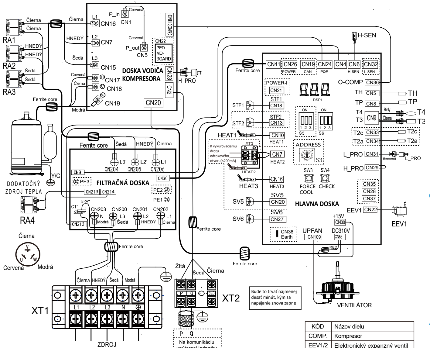
Obrázok 4-3.1: HOP12(14,16)WODU3, schéma zapojenia
